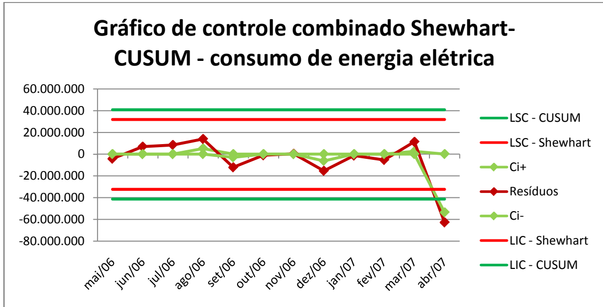
Figura 28 - Gráfico de controle combinado Shewhart-CUSUM com parâmetros K = 0,5 , H = 2,3 e LS = 1,8 , aplicado aos resíduos do modelo de previsão para o consumo industrial de energia elétrica em Santa Catarina
