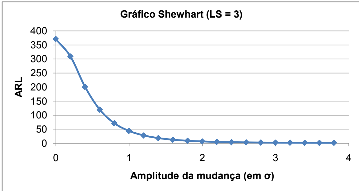
Figura 5 - Curva de desempenho do gráfico de controle de Shewhart para diferentes amplitudes de mudança (em \sigma ) no processo Fonte: Software de simulação, Rocha (2004)
