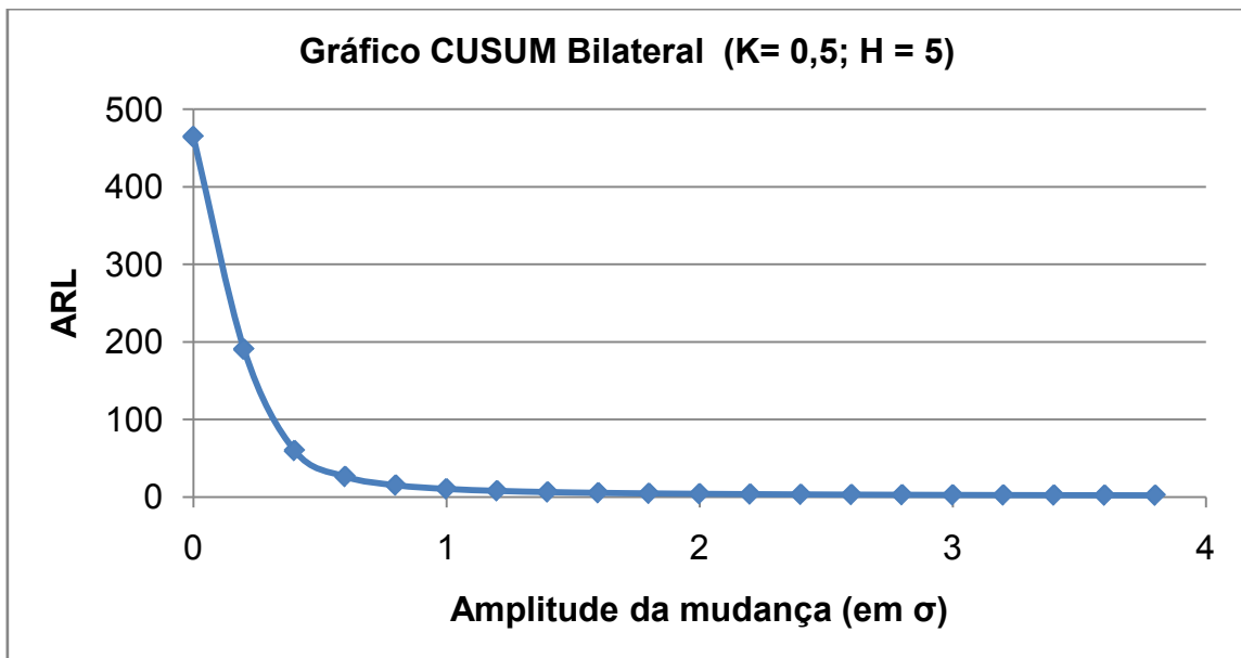
Figura 6 - Curva de desempenho do gráfico de controle CUSUM para diferentes amplitudes de mudança (em \sigma ) no processo Fonte: Software de simulação, Rocha (2004)
