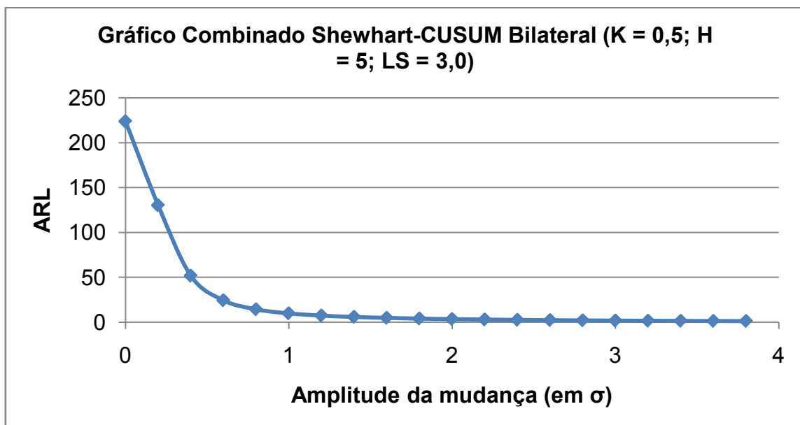
Figura 8 - Curva de desempenho do gráfico de controle combinado Shewhart-CUSUM (LS = 3,0) para diferentes amplitudes de mudança (em \sigma ) no processo Fonte: Software de simulação, Rocha (2004)
